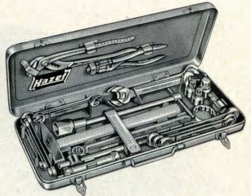
Kastengröße: 450 × 200 × 55 mm
